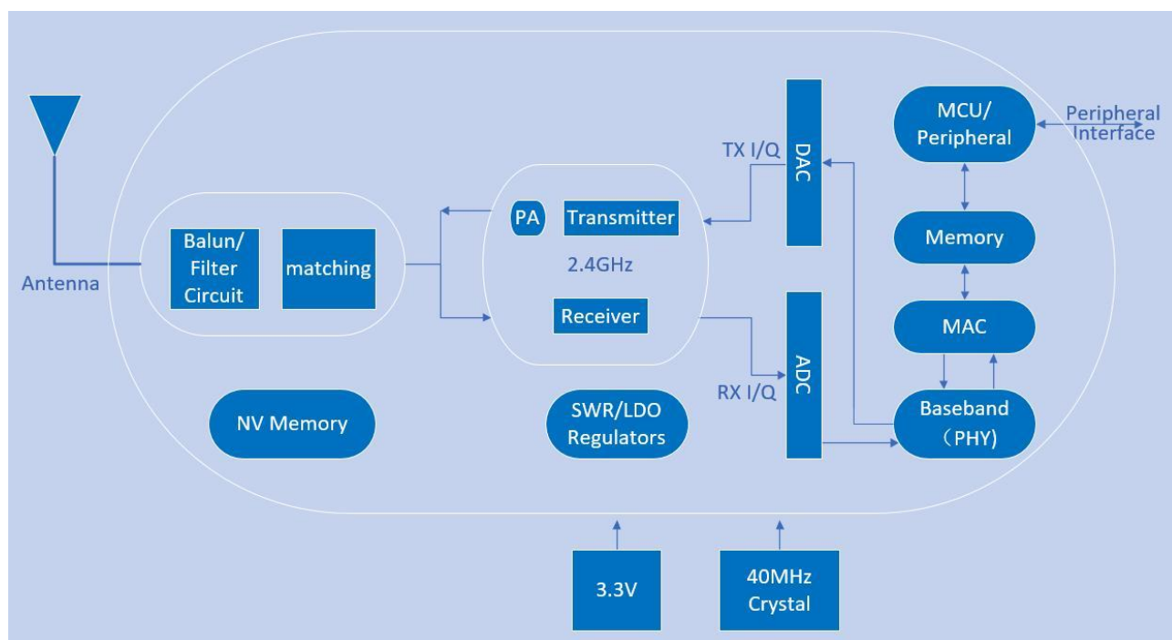
图 1 模块框架
